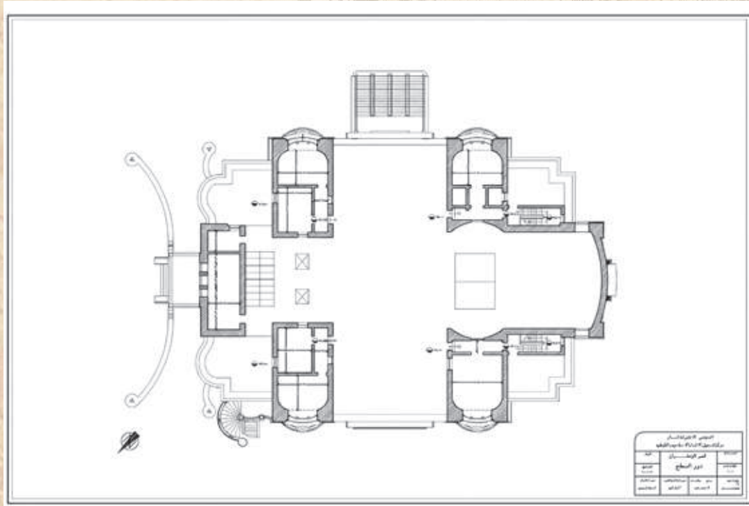
شكل ٣١: تخطيط دور السطح لقصر الزعفران
