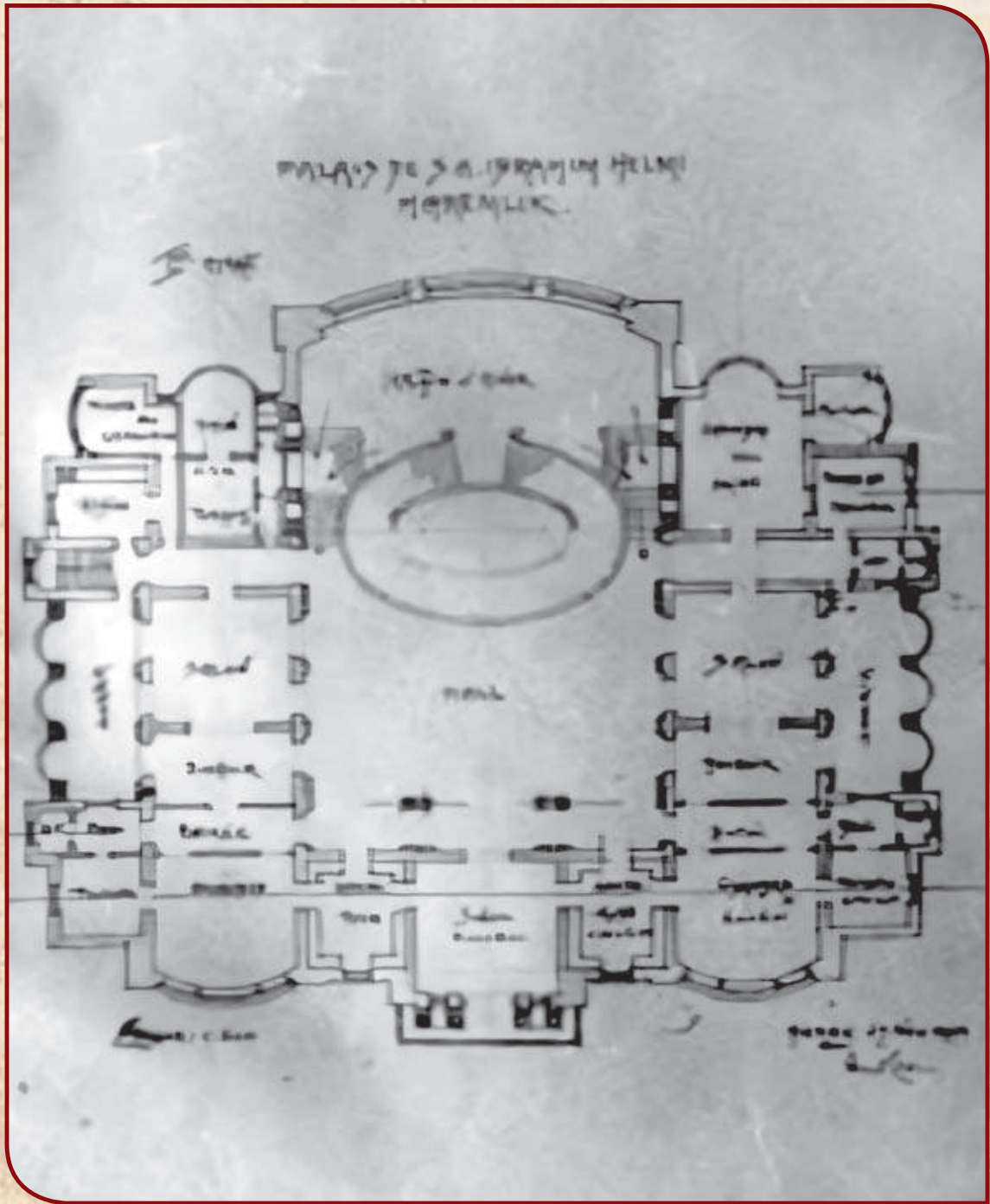
شكل ٢١: تخطيط الدور الأول لقصر الزعفران الذي عرضه لاشياك على إبراهيم حلمي باشا ابن جناتيار هانم واحدة من صاحباتي القصر؛ عن: Kuzmin, Lasciac, p. 113 fig. 63.
