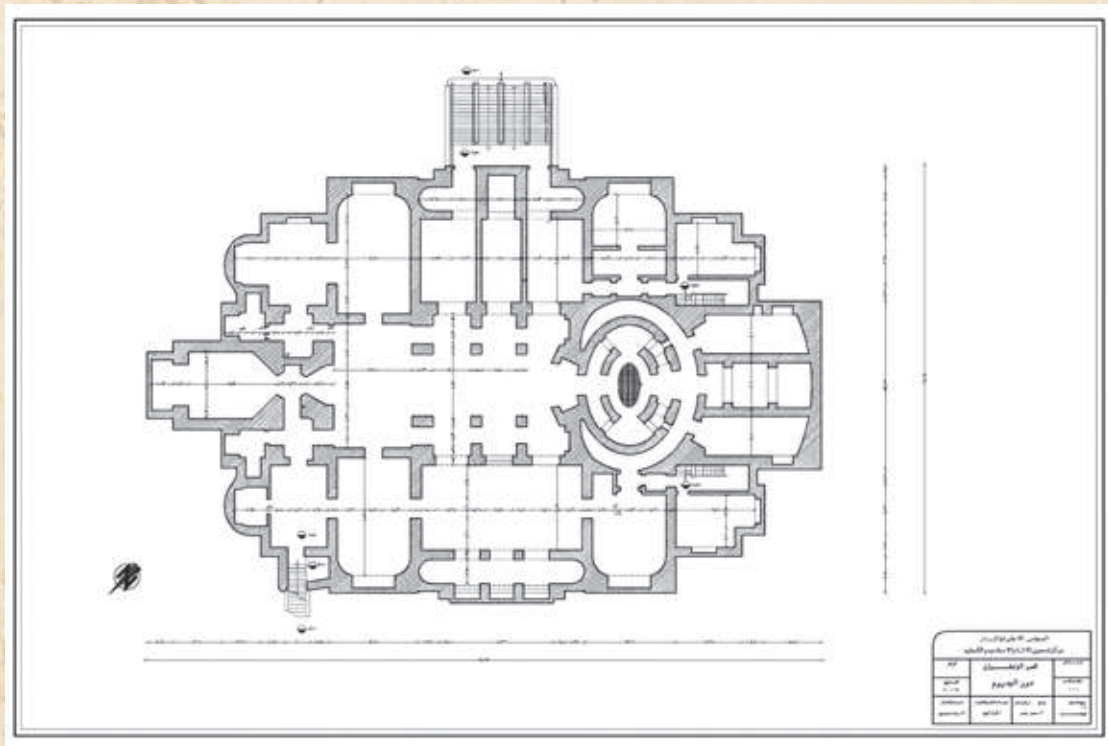
شكل ٣٠: تخطيط دور البدروم لقصر الزعفران
